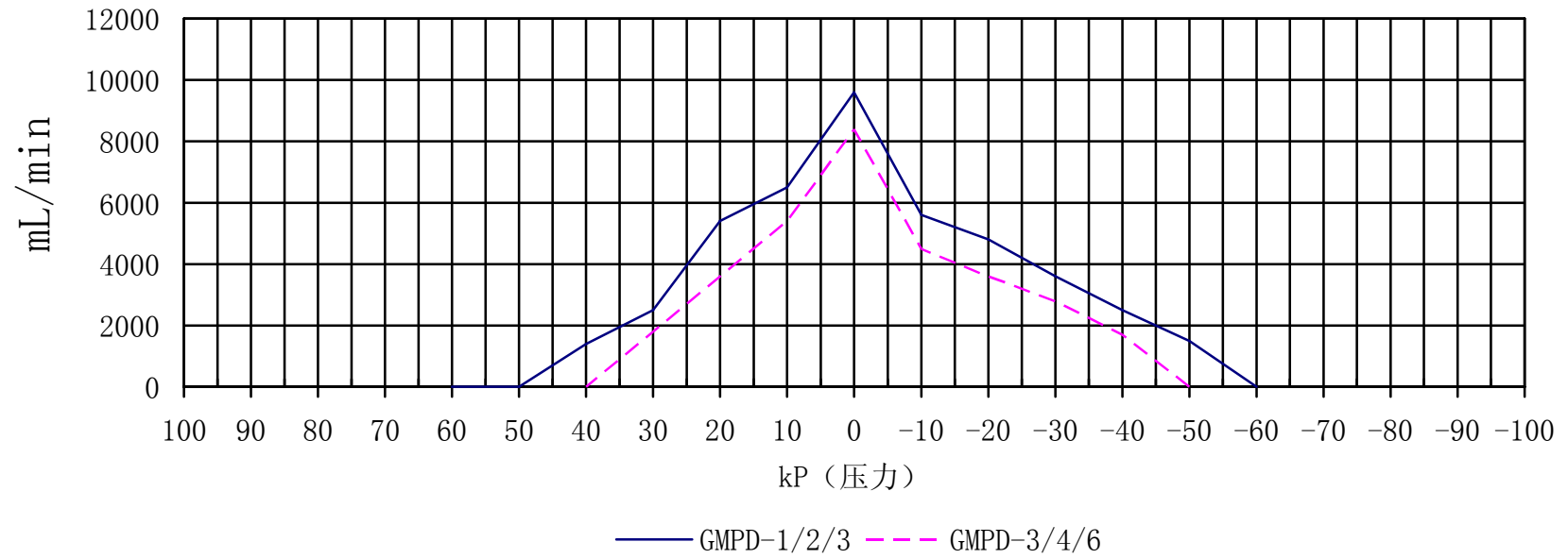
GMPD系列流量负载图
